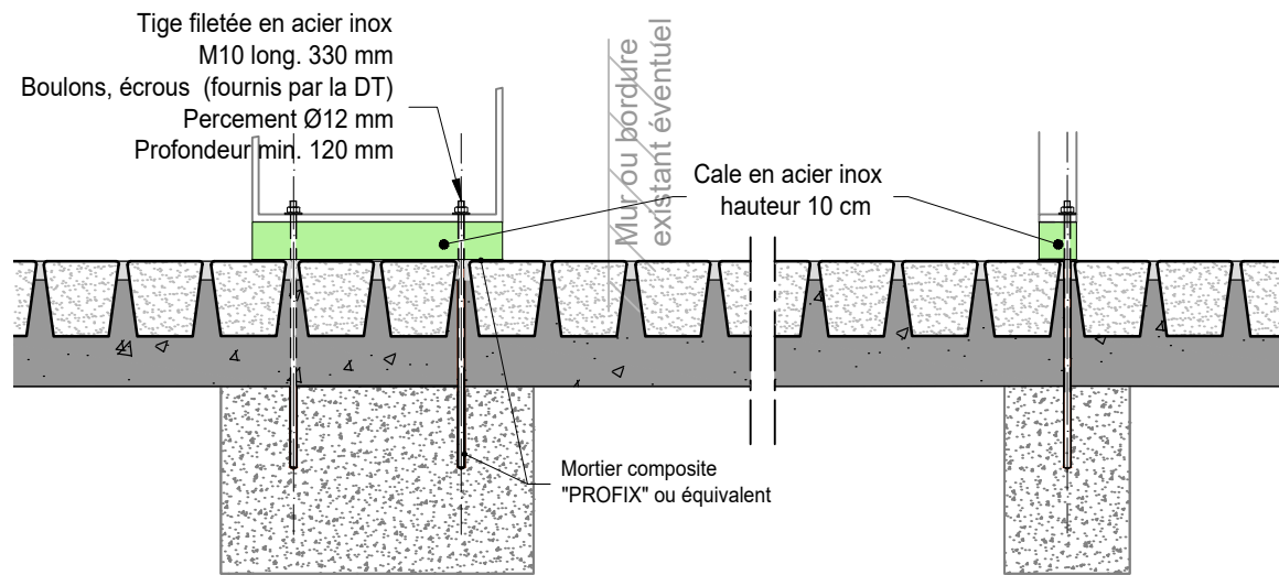
Détail de fixation
