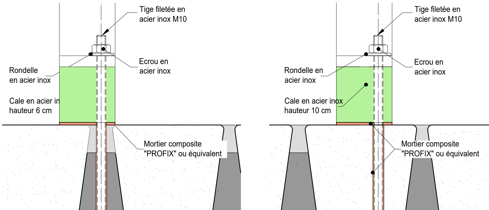
Dans le joint
